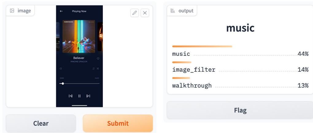
Figura 20 Interfaz que obtiene baja confianza.
