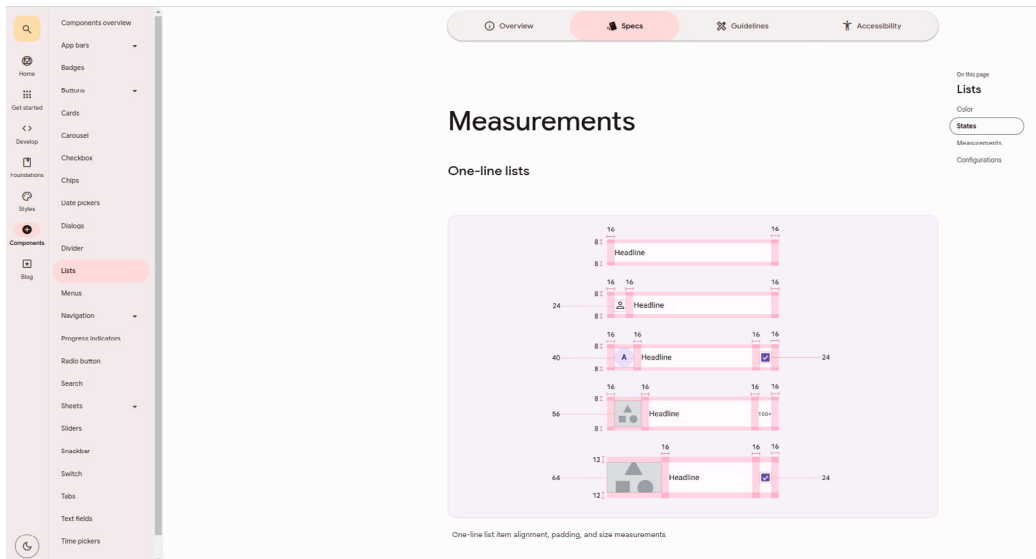
Figura 5. Medidas o tamaños de los elementos del componente list, expresado en píxeles, generalmente múltiplos de 8 (Material Design 3, 2021e).
