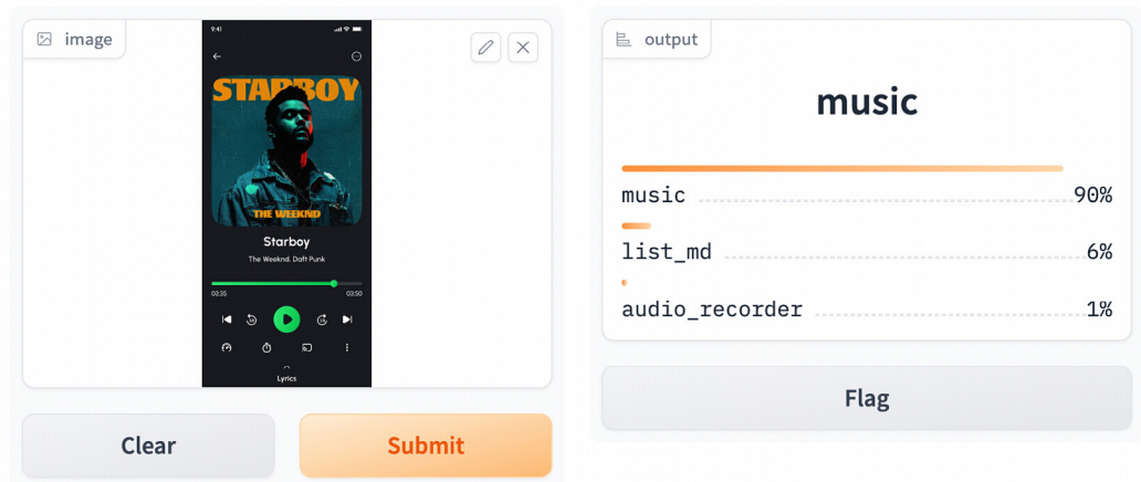
Figura 19. Interfaz que obtiene alta confianza.
